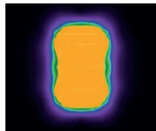
LO: Beleuchtung eines Sportplatzes mit Scheinwerfern mit Streulichtbegrenzung (LO)
