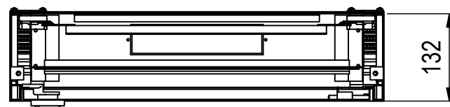
B-B ( 1 : 8 )
