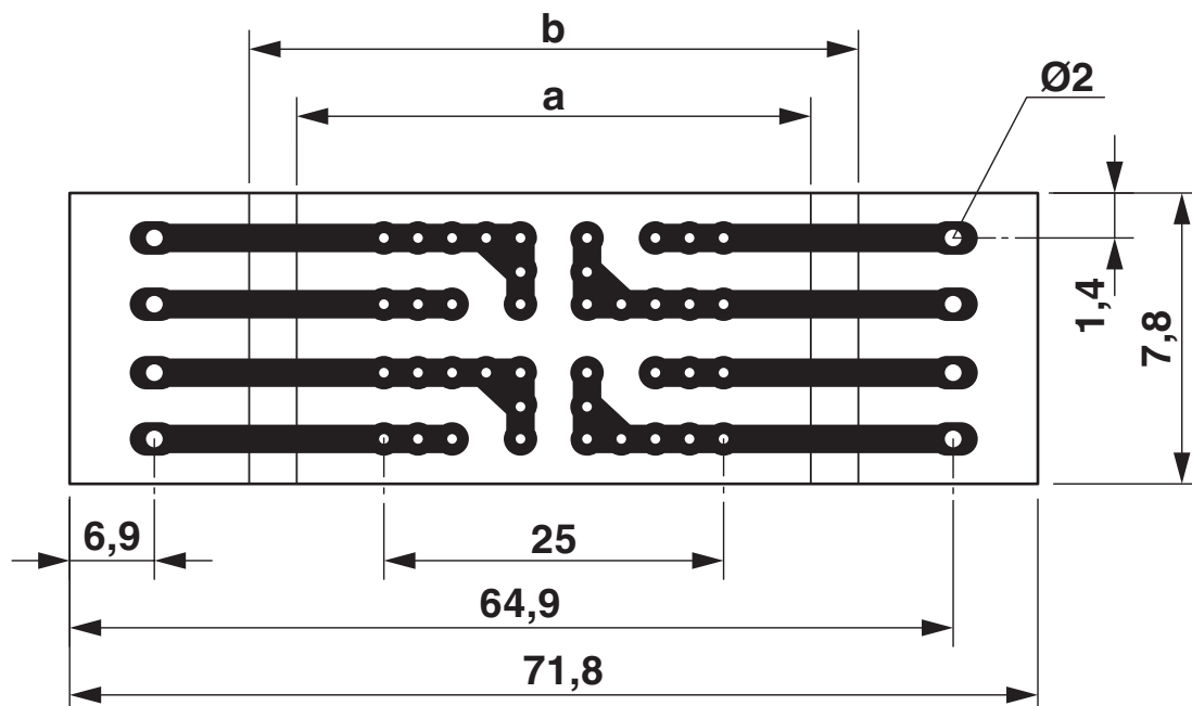
Maßzeichnung
