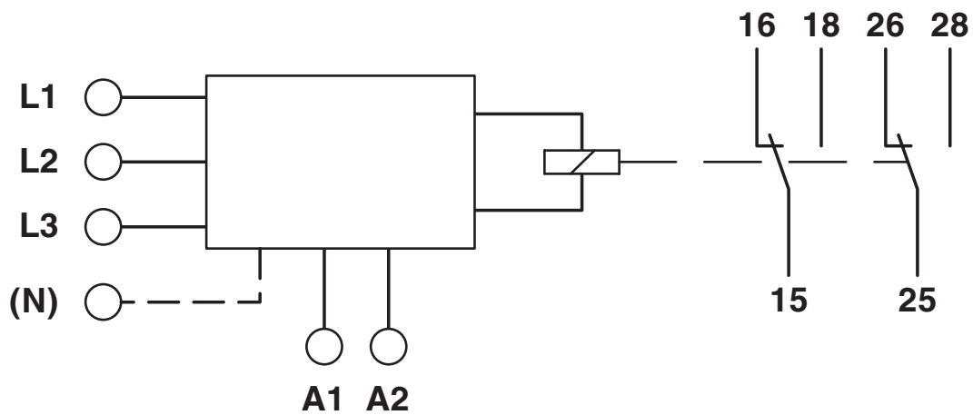
Blockschaltbild
