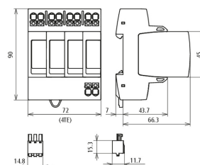
Maßbild DG SMP TNS 275 FM
