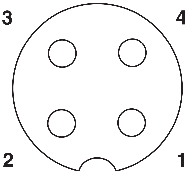
Polbild Buchse M12, 4-polig, A-kodiert, Ansicht Buchsenseite
