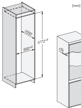
KFN7714F, KFNS7716FC, Einbau (Fußnote*) (Skizze)
