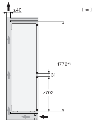
KFN7714F, KFNS7716FC, Seitenansicht (Skizze)
