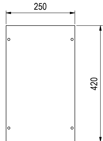
Montageplatte ( 1 : 7 )
