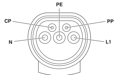
Pinbelegung Fahrzeug-Ladestecker
