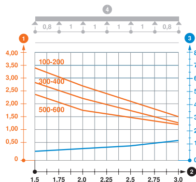
Belastungsdiagramm Kabelrinne Typ SKSM 85
