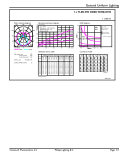
LEDtube 8W G13 850lm 830
