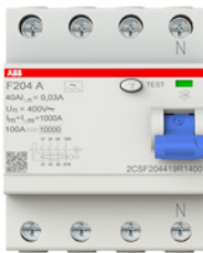
FI-Schutzschalter Typ TG
