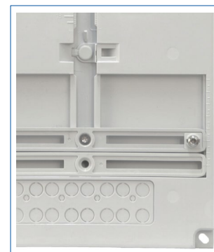
Detail Plombierkappe und zweite Befestigungsschiene
