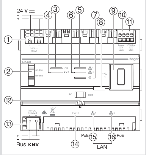
Bild 1: Aufbau des Geräts
