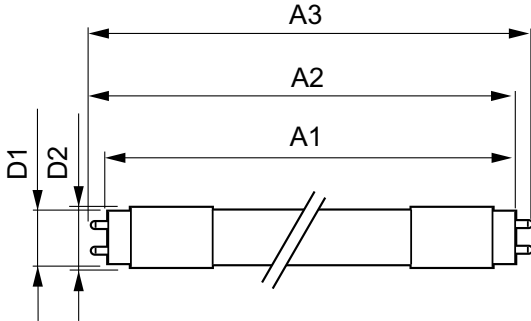
TLED 1200mm UNV16W-36W 2100lm 6500K
