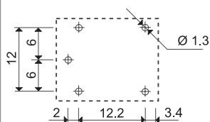
Ansicht auf die Anschlüsse
