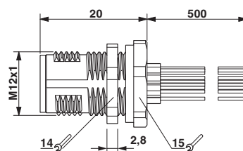
Maßzeichnung
