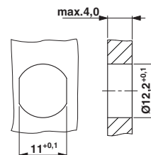
Maßzeichnung
