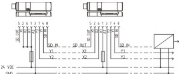
Schaltungsbeispiel
