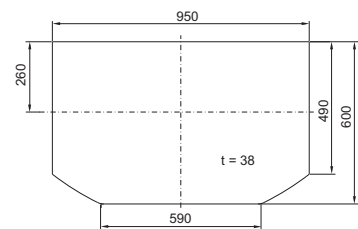
Arbeitsplatte, vorbereitet für Standfuß IW 6902.310
