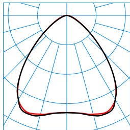
Mirona Fit 2L B 130-840 ETDD ESG TX050467
