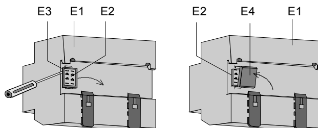
Bild 4: Abdecken des Kontaktsystems
