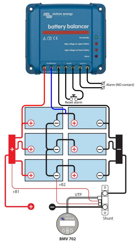
Battery Balancer, der am sechs in Serie geschaltete 12 V Batterien (24 V-System) angeschlossen ist.
