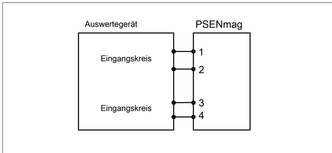
Abb.: Zweikanaliger Anschluss des PSEN ma1.4a-50 an den Eingangskreisen eines Auswertegeräts
