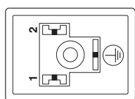
Polbild Ventilstecker, Bauform B
