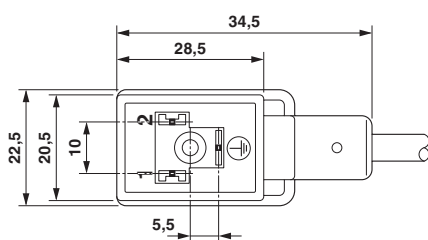
Ventilstecker, Bauform B
