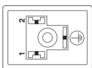
Polbild Ventilstecker, Bauform B
