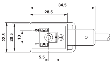
Ventilstecker, Bauform B
