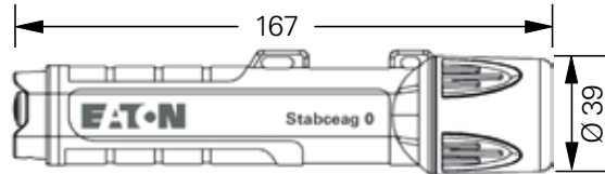
Maßzeichnung Stabceag 0
