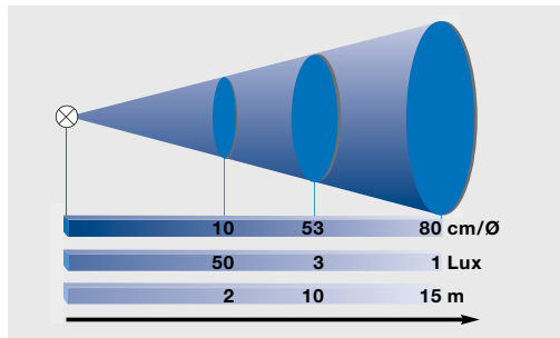
Reichweiten-Diagramm Stabex HF-LED
