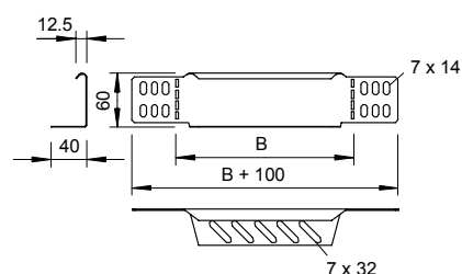
Abmessungen
