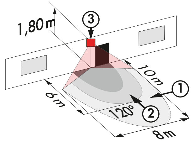
Reichweitendiagramm
