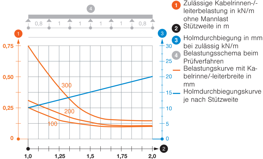
Belastungsdiagramm Gitterrinne GR-Magic Typ GRM 35
