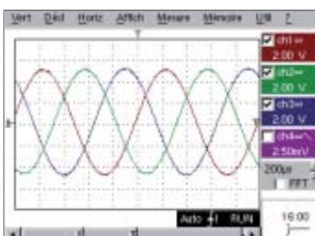
Beispiel 1, Simulation eines Drehstrom-Signals
