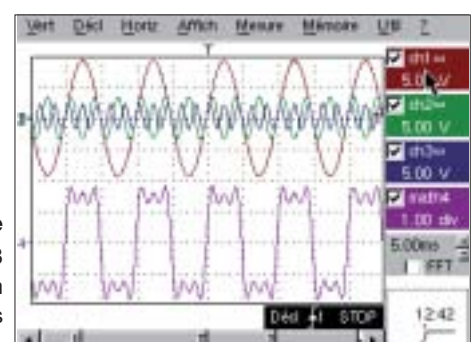
Beispiel 1, Simulation eines Drehstrom-Signals
