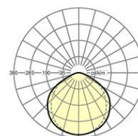
Lichttechnik freistrahlend-direkt freistrahlend SDGV LED 4200 lm 840
