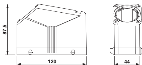
Maßzeichnung
