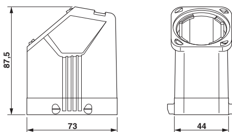
Maßzeichnung
