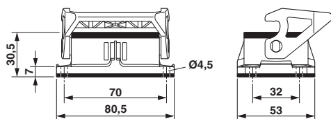
Maßzeichnung
