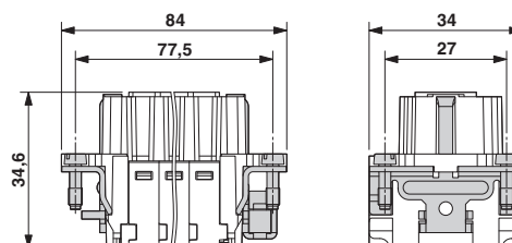
Buchseneinsatz
