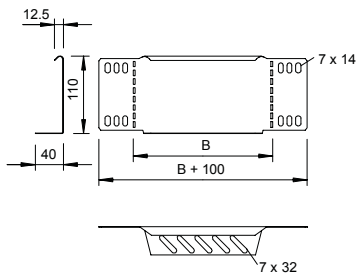
Abmessungen
