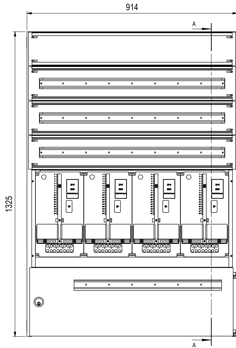
Hutschiene Vorzählerfach 839
