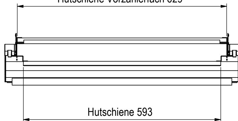
Hutschiene Vorzählerfach 629
