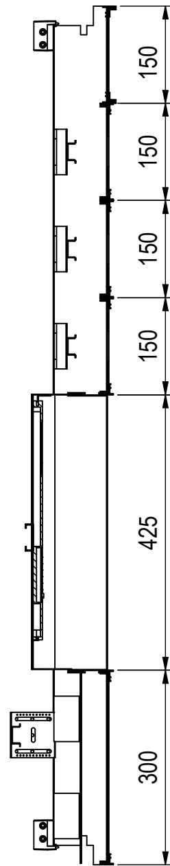
A-A (1:8)
