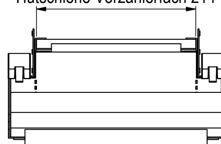
Hutschiene Vorzählerfach 214
