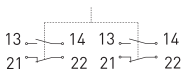
Schaltbild
