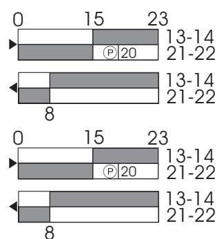
Schaltwegdiagramm
