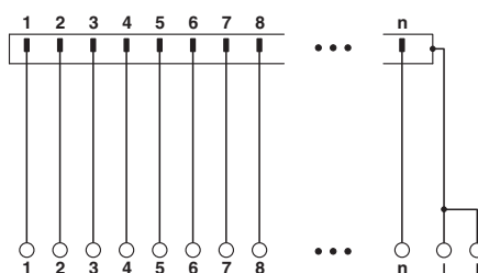
Schaltplan
