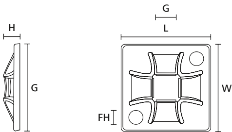
Q-Mount (Seitenansicht)
