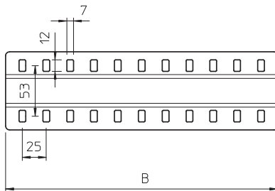
Abmessungen
