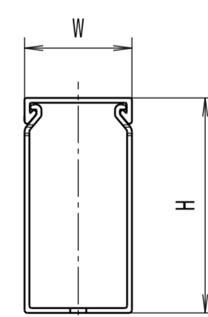
Montagezustand mit Deckel/ Assembly condition with cover
