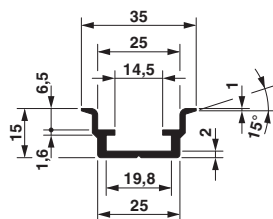
Maßzeichnung
