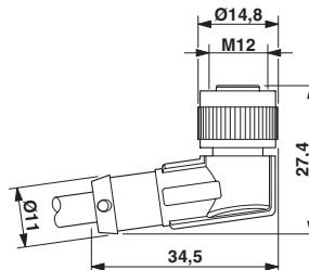
Maßzeichnung
