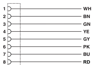
Schaltplan
