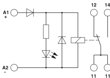
Schaltplan
