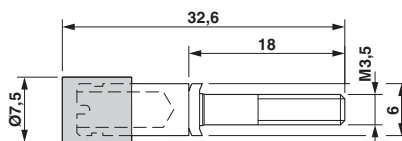
Maßzeichnung
